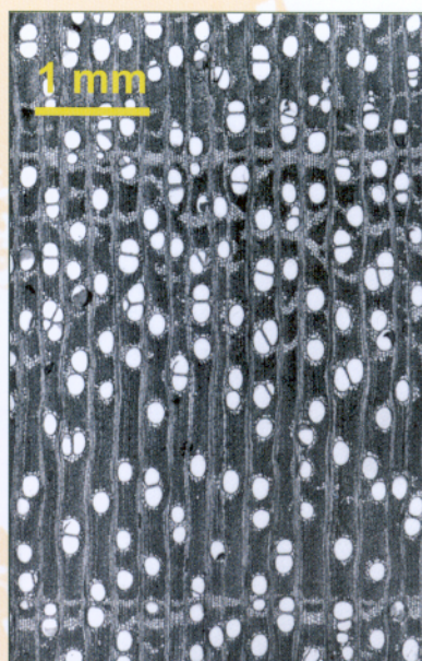
Section transversale du bois du sapelli. Crad-forêt
