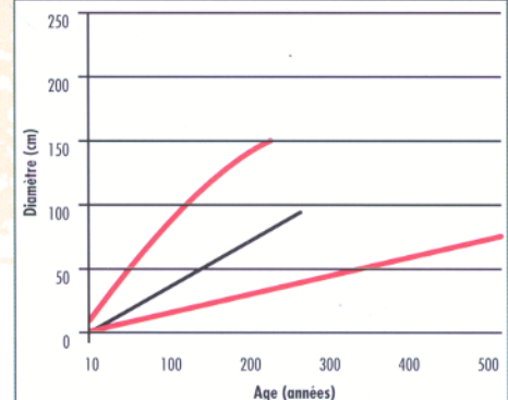
Figure 4. Limites supérieures et inférieures de croissance observées par l'analyse de cernes sur 104 sapellis à Sangha Mbaéré, République centrafricaine. B. Demarquez
